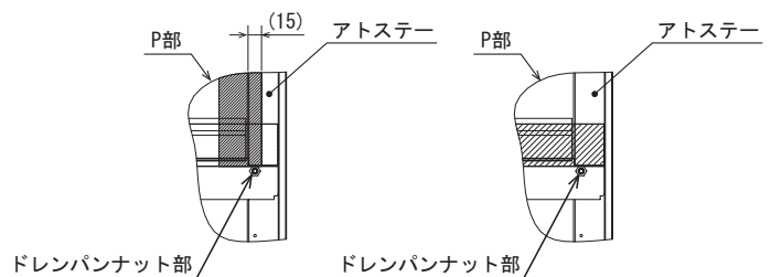
1. 断熱材(小)貼付図
