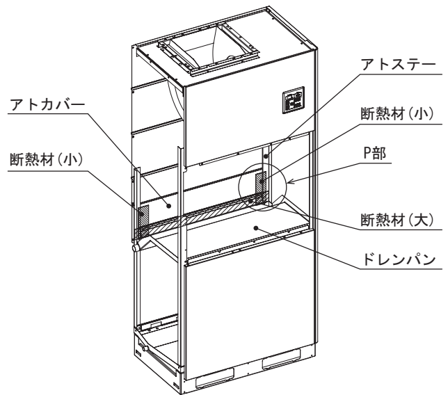
1. 断熱材(小)貼付図
