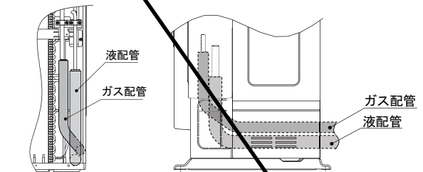
室外ユニット正面より 室外ユニット右側面より
