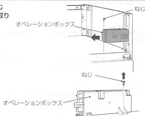
オペレーションボックスを裏から見た図
