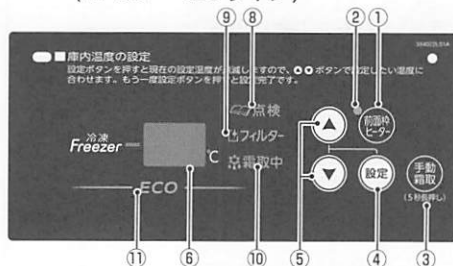
(HF-150 ~ 180 タイプ)
